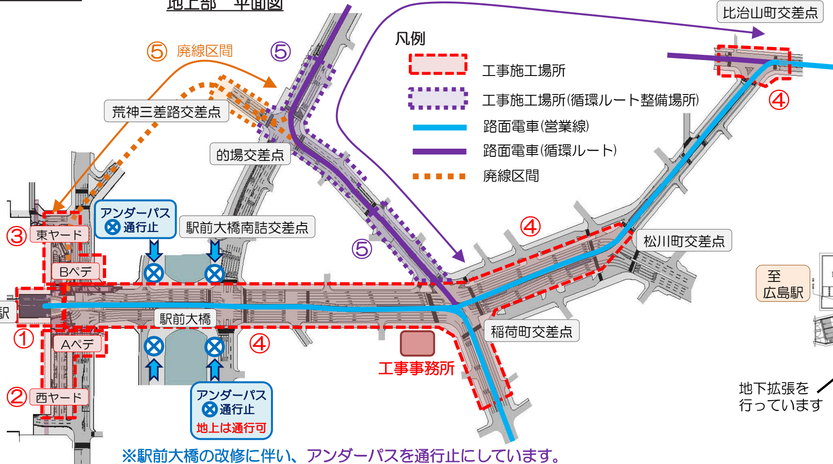
地上部 平面図
